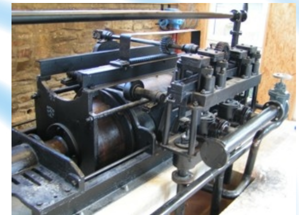
Lambach-Pumpe (Wassersäulenmaschine)
